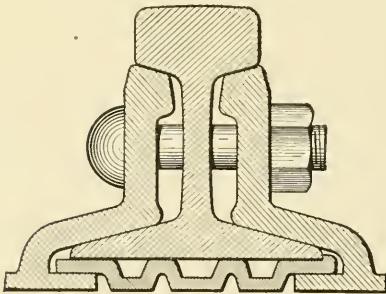
Fig. 228. Wolhaupter Joint
